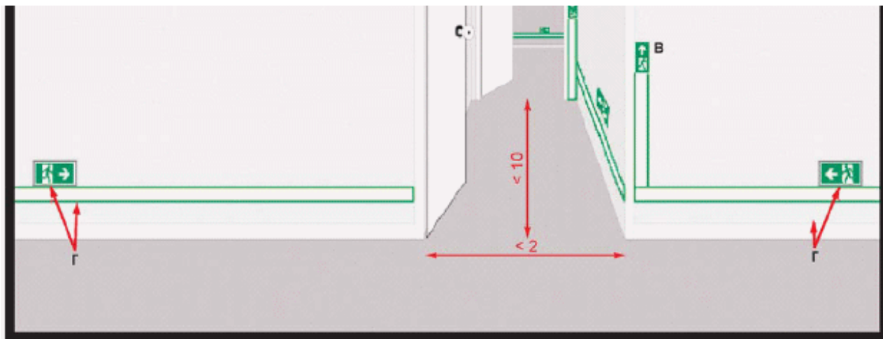
Рисунок А.3 - Примерный план Т-образного перекрестка, ведущего в прямой коридор (с более чем одной дверью), показывающий непрерывность обозначения
