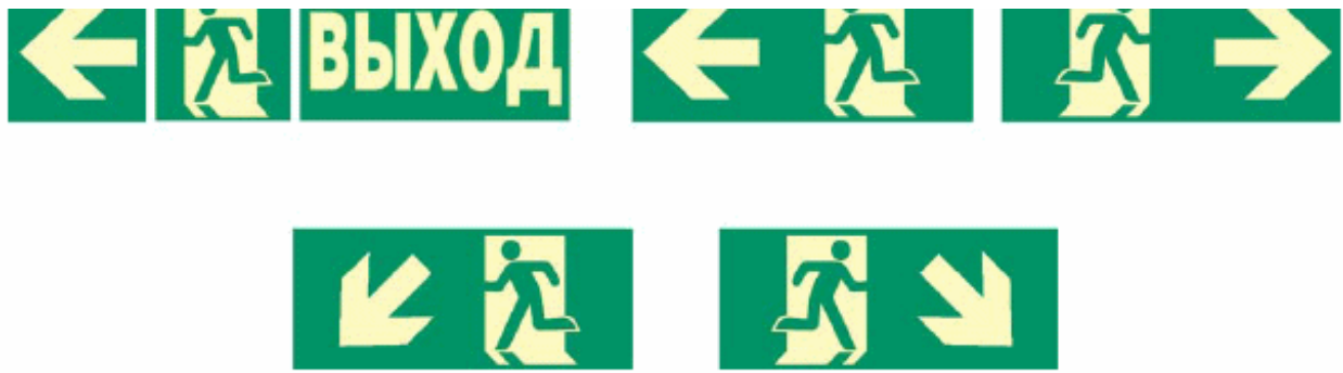
Рисунок 2 - Примеры знаков маршрутов эвакуации или указателей направления, которые допускается использовать вместе с текстом
