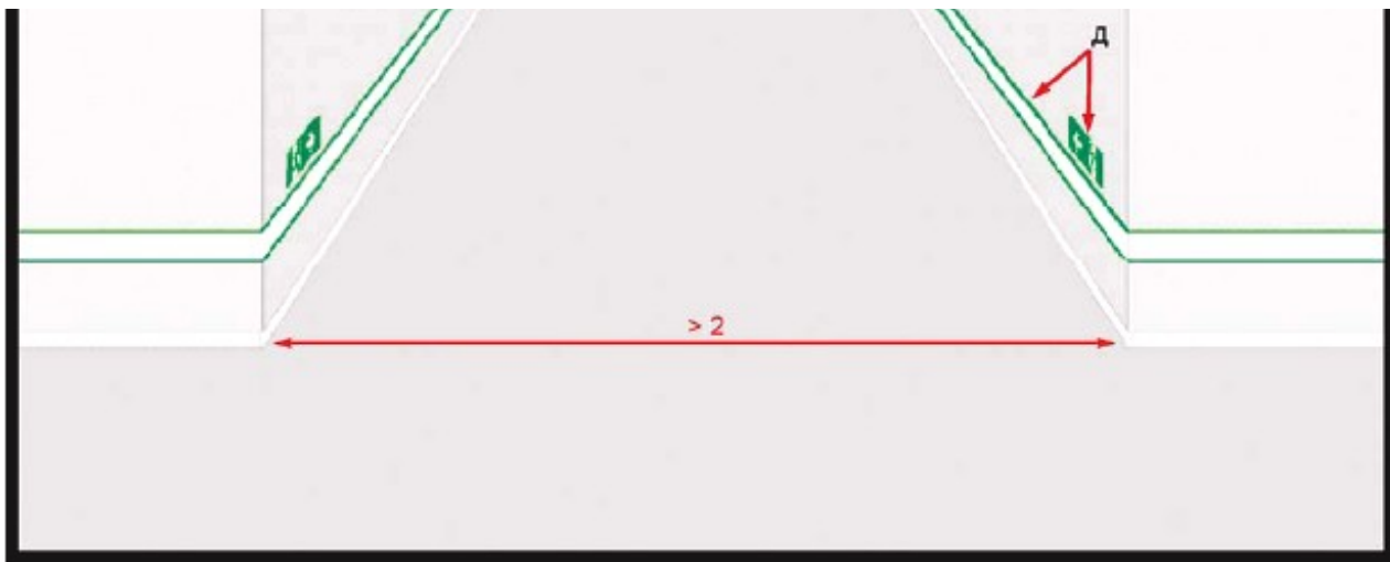
Рисунок А.2 - Примерный план коридора шириной более 2 м с низкорасположенными направляющими линиями с обеих сторон
